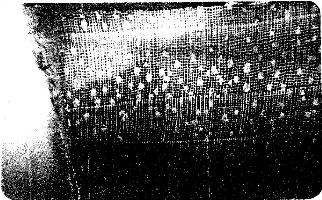
Fig.8 Macroscopía, corte transversal (8x), muestra radios medulares, poros y parénquima apotraqueal en bandas.
